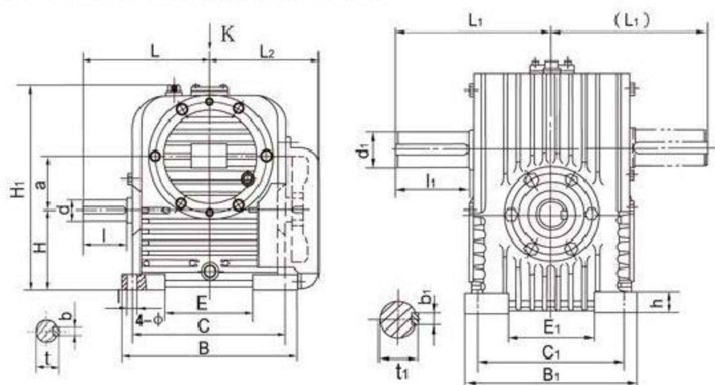
TPU型减速器（整箱式）及装配型式
