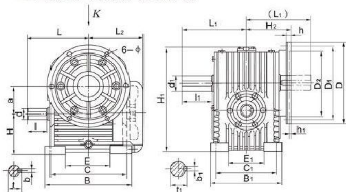
TPS型减速器（整箱式）及装配型式
